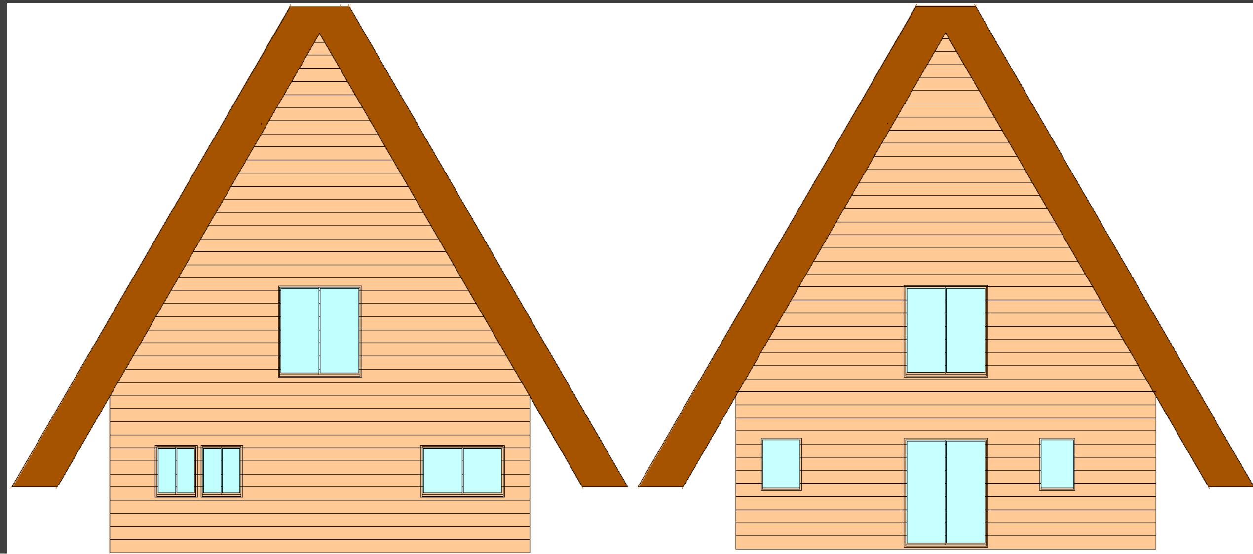
西立面图
