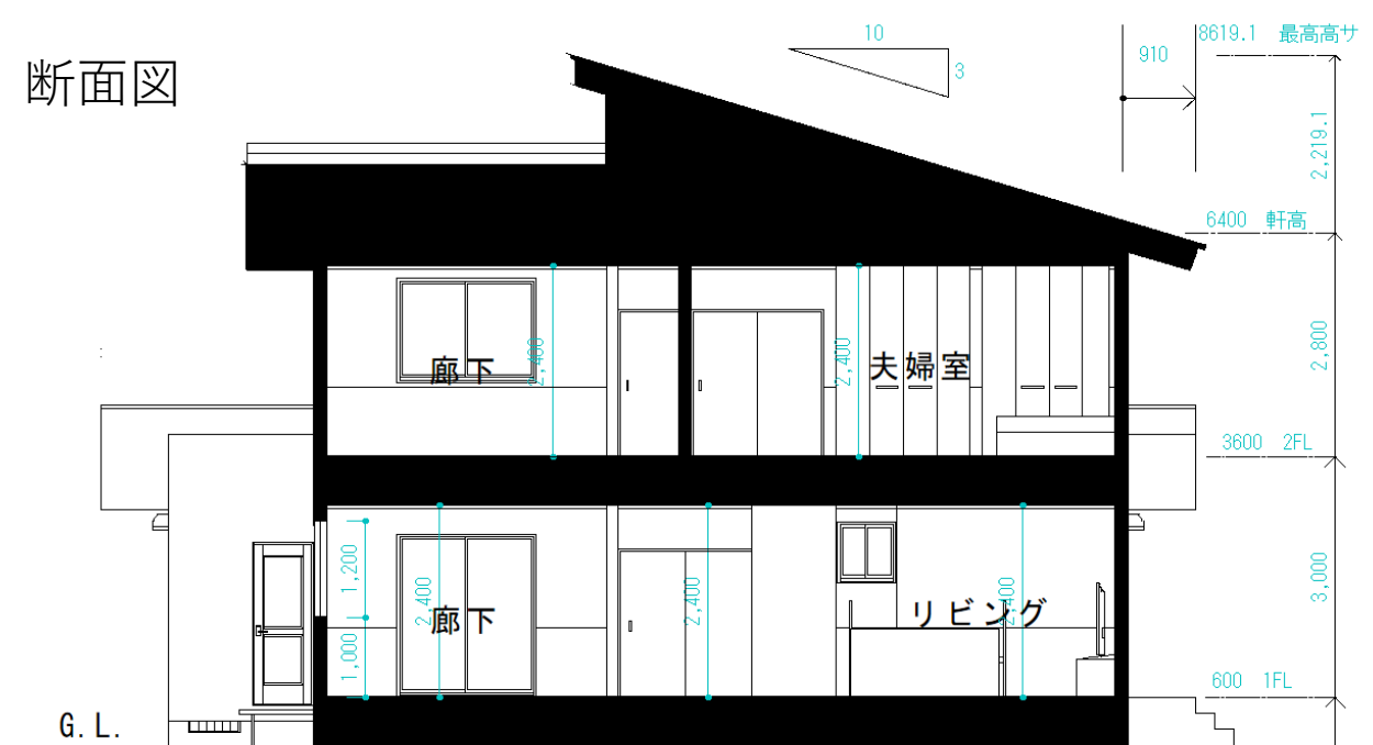
南立面図
