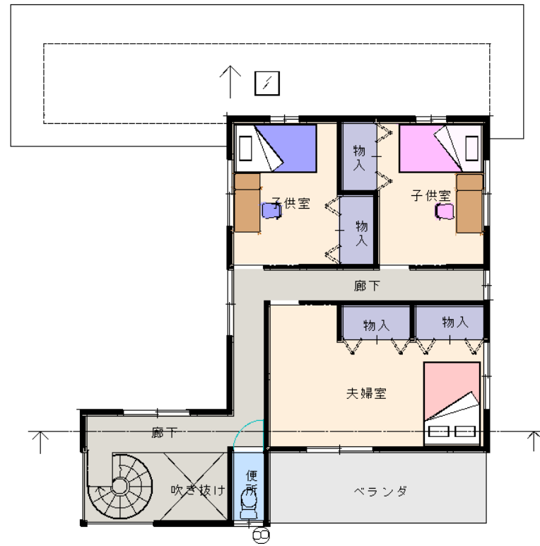
2階平面図
