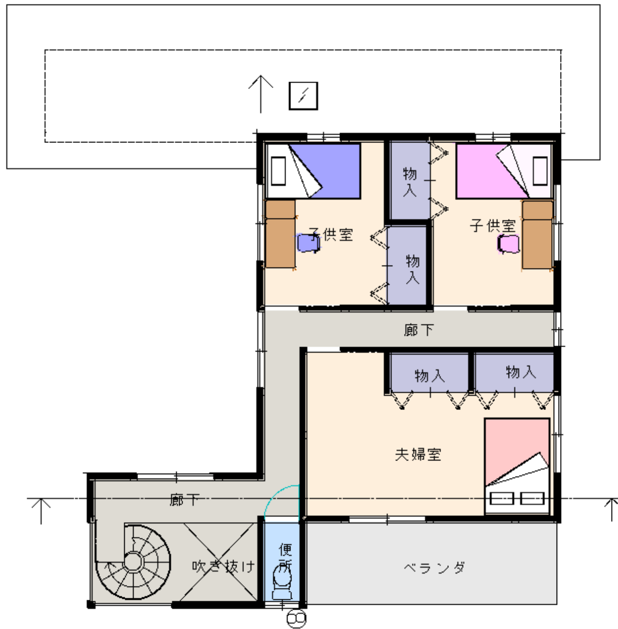
2階平面図
